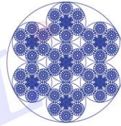
6X[6X64SFS+IWR]+IWRC
