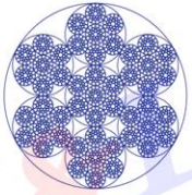
6X[6X36WS+IWR]+IWRC
