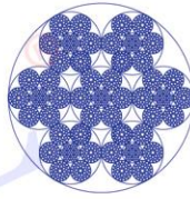
6X[6X55SWS+IWR]+IWRC
