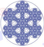
6X[6X41WS+IWR]+IWRC
