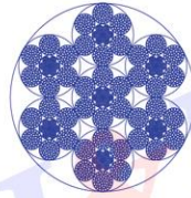
6X[6X61FWS+IWR]+IWRC
