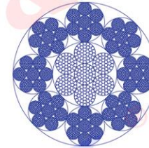
8X[6X61+IWR]+IWRC
