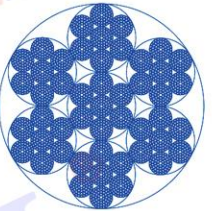
6X[6X61+IWR]+IWRC
