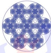
6X[6X49SWS+IWR]+IWRC
