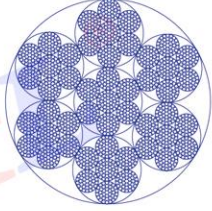
6X[6X37+IWR]+IWRC
